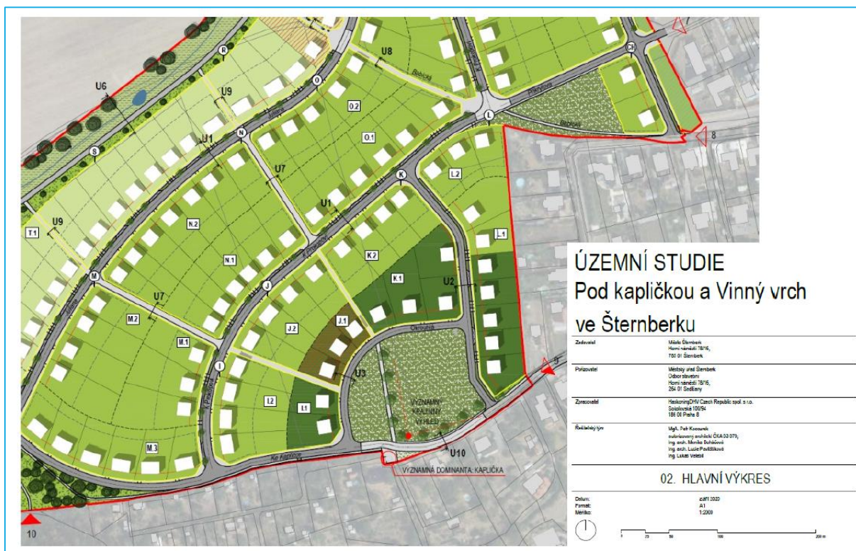
Územní studie Pod kapličkou a Vinný vrch ve Šternberku – výřez z hlavního výkresu
