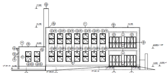
DDM příprava PD na rekonstrukci – obálka budovy B („zelená střecha“, zateplení fasády vč. výměny otvorů)
